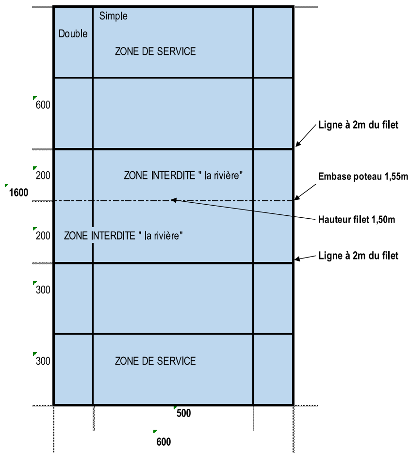
DIMENSIONS DU TERRAIN en DALLES EXTERIEURES
